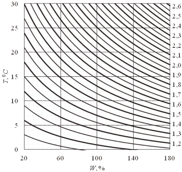
Рис. 1. Номограмма для определения поправочного коэффициента a_{WT} на совместное влияние температуры и влажности древесины сосны при расчете удельной работы резания при поперечном пилении цепями
