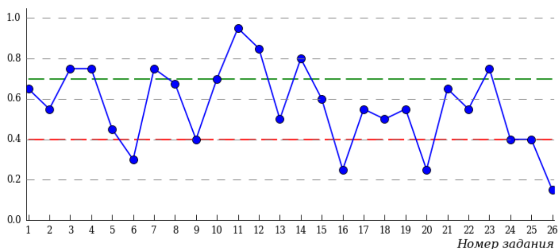
Коэффициент решаемости
