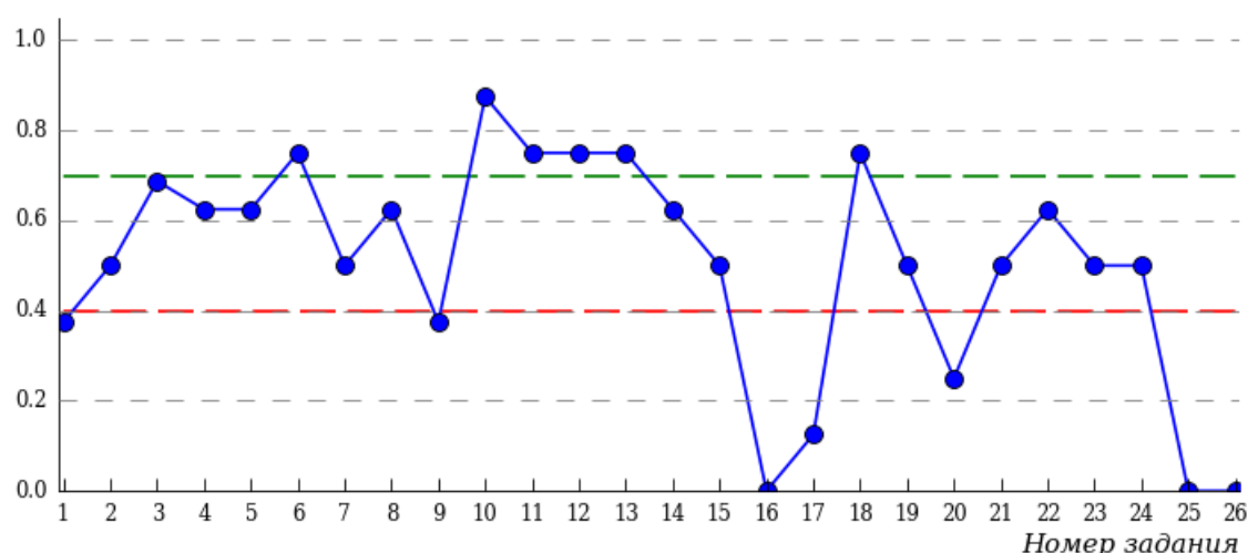
Коэффициент решаемости
